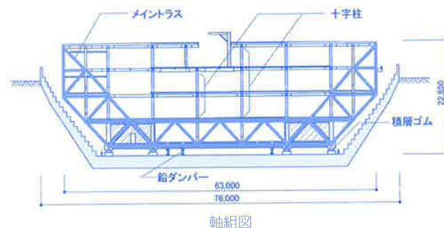
軸組図
