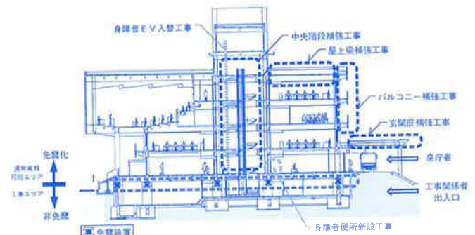
改修工事概要(断面図)
