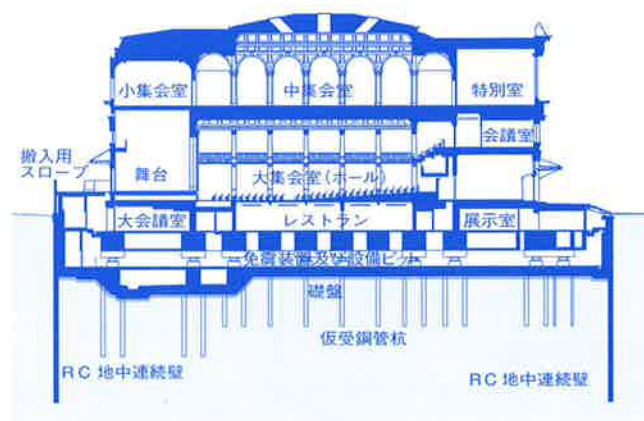
断面図
