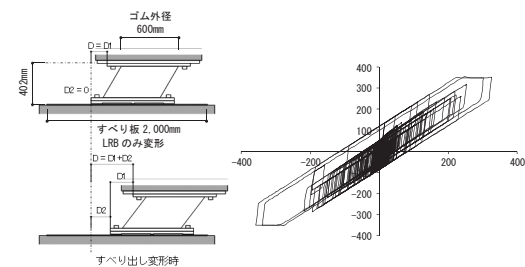
図23 QTBの変位－水平力関係
