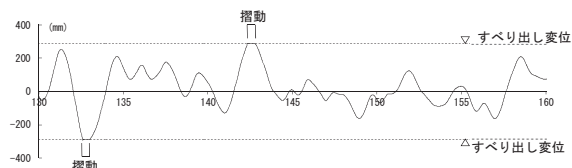
図22 D1の時刻歴変化
