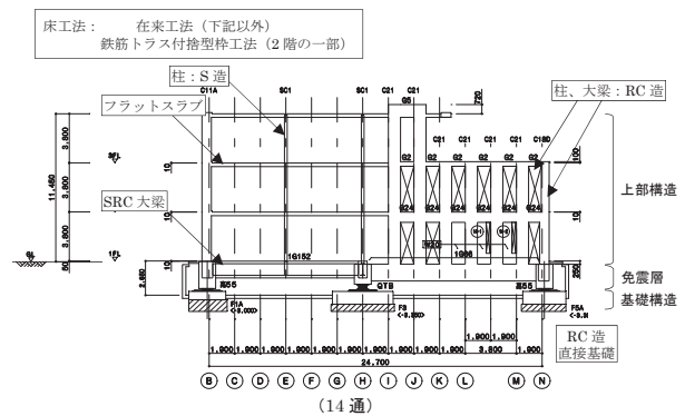
図7 構造計画概要図 (2)
