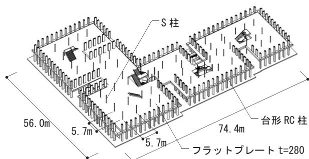
図9 基準階構造体アクソメ
