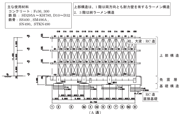
図6 構造計画概要図 (1)
